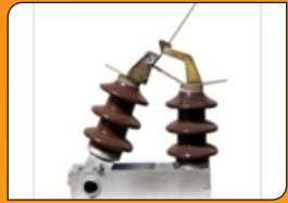
JTS 001 - 11 KV SP AB SWITCH
